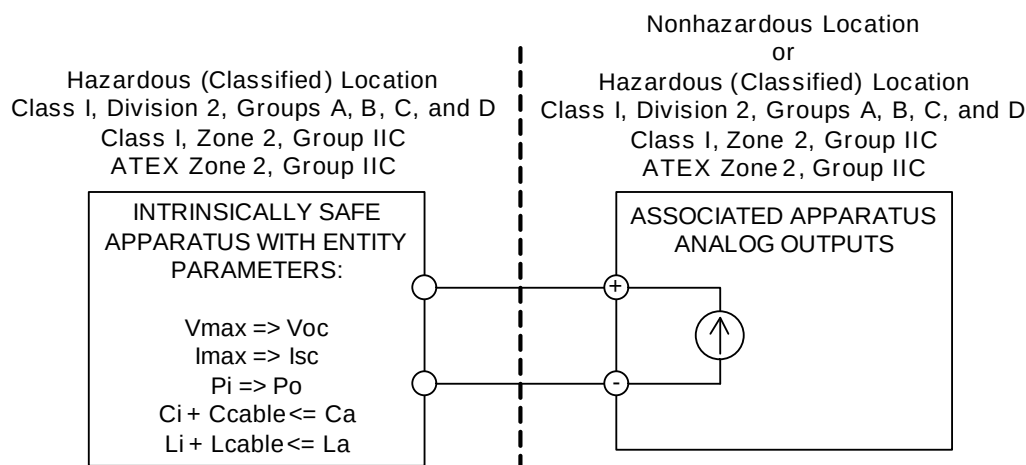
Entity Parameters
