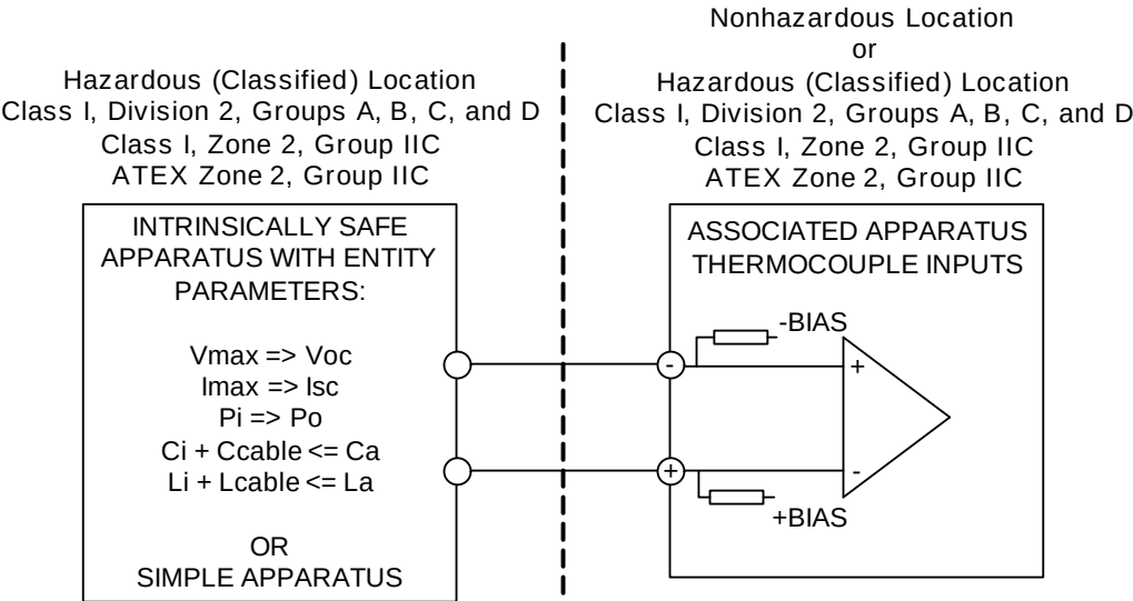
Entity Parameters
