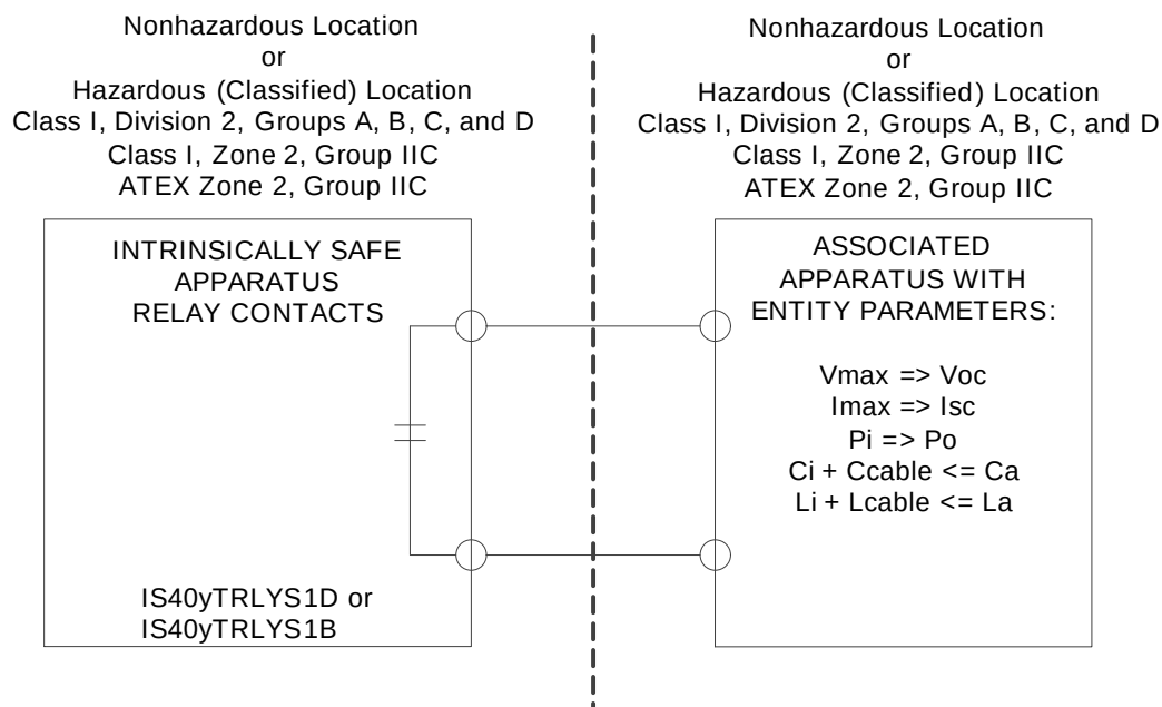
Entity Parameters
