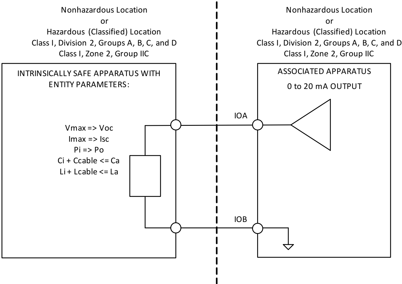
Entity Parameters
