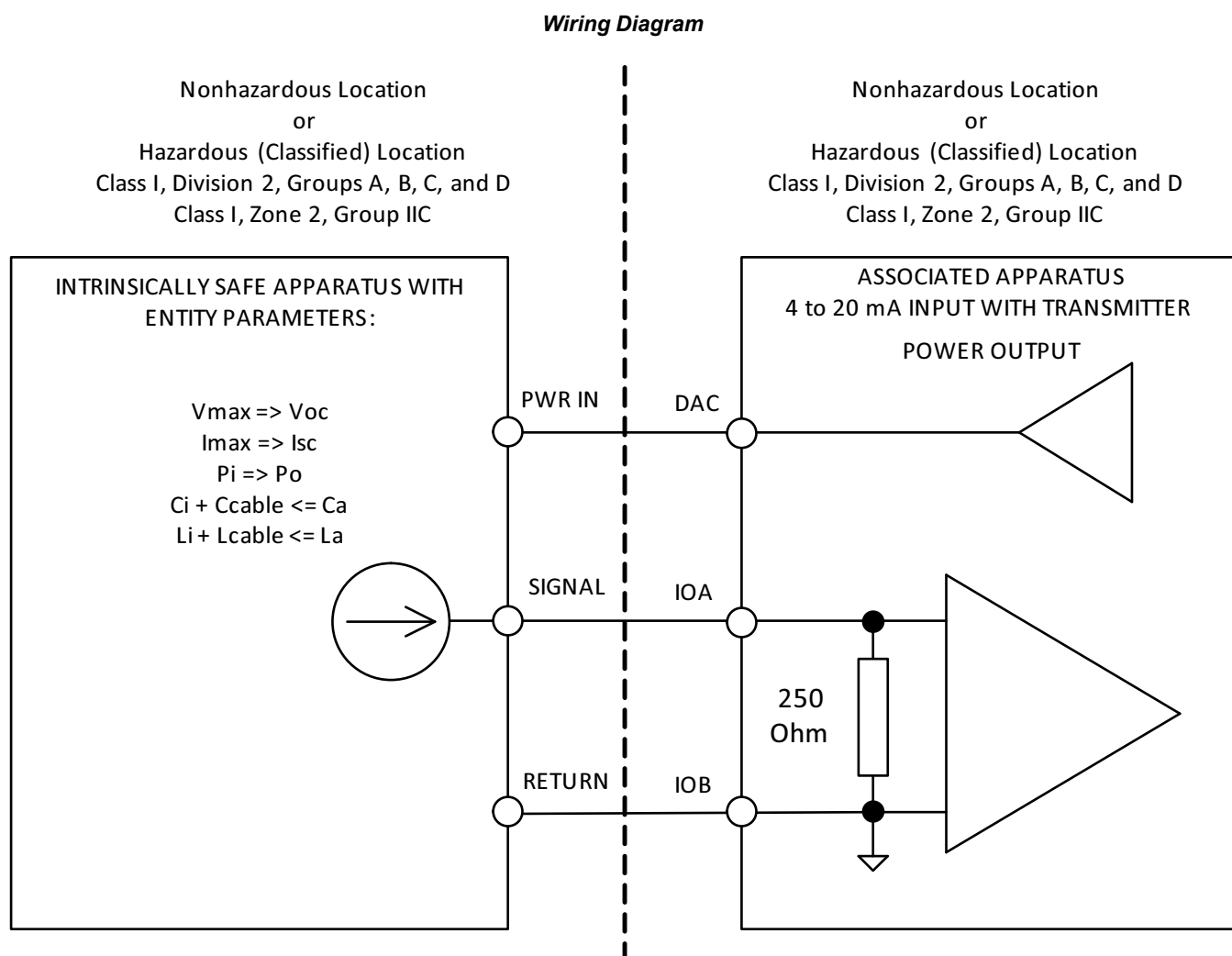
Entity Parameters
