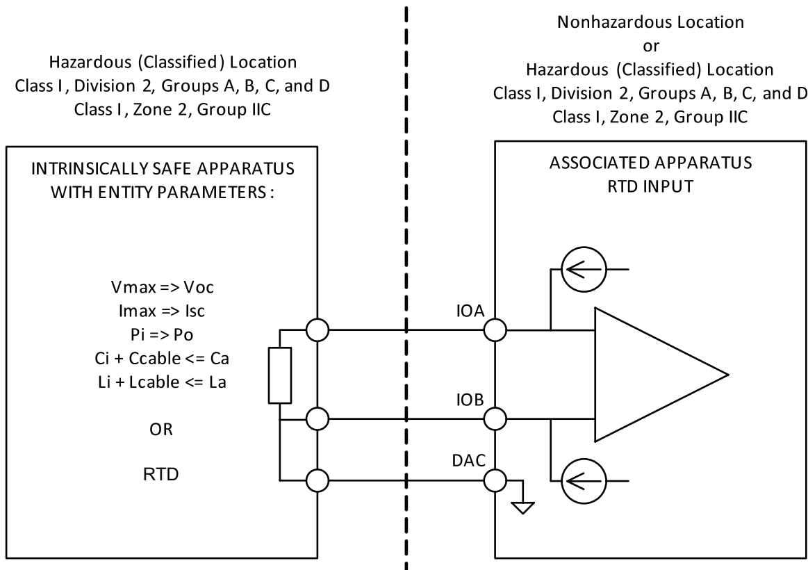
Entity Parameters
