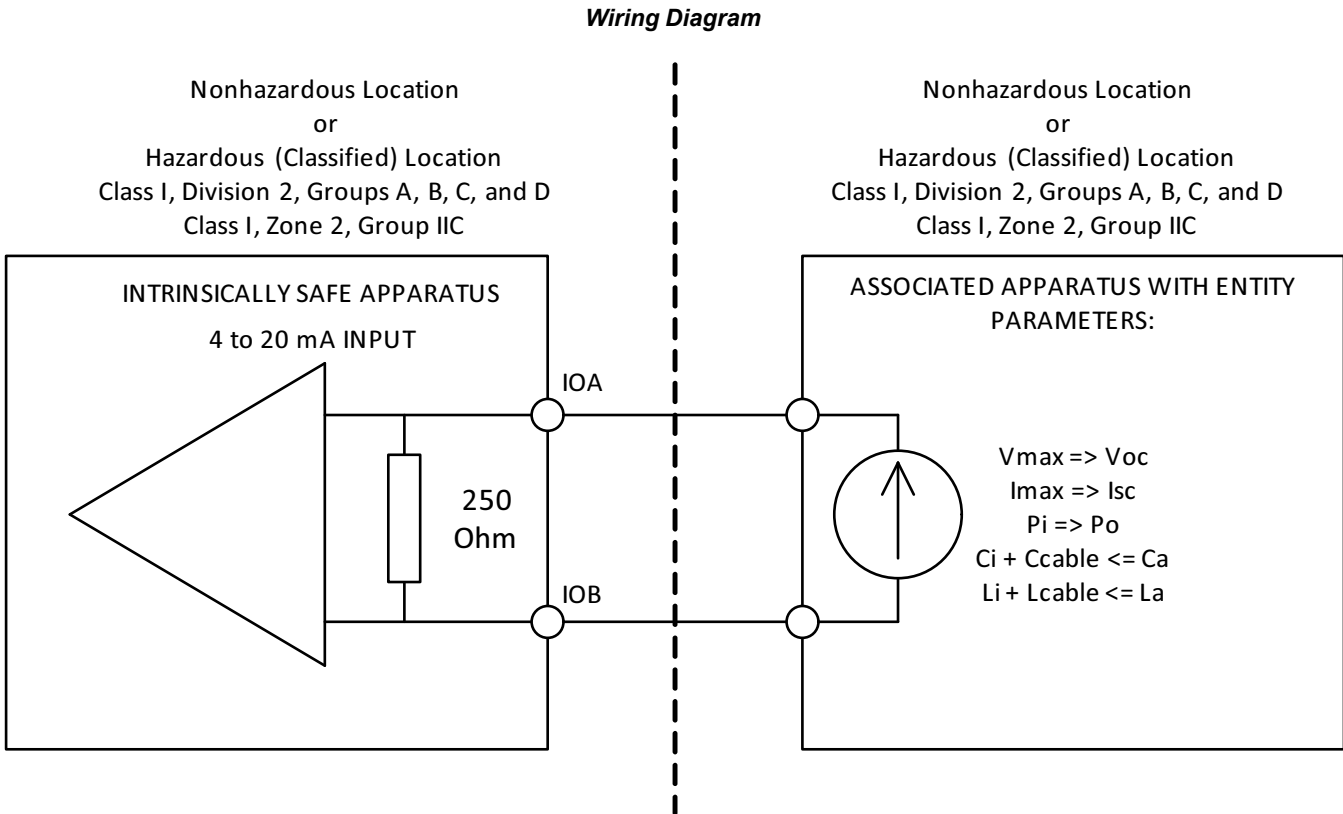
Input Parameters
