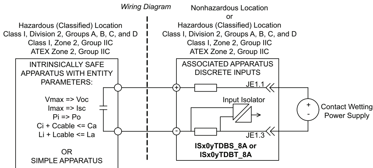
Entity Parameters
