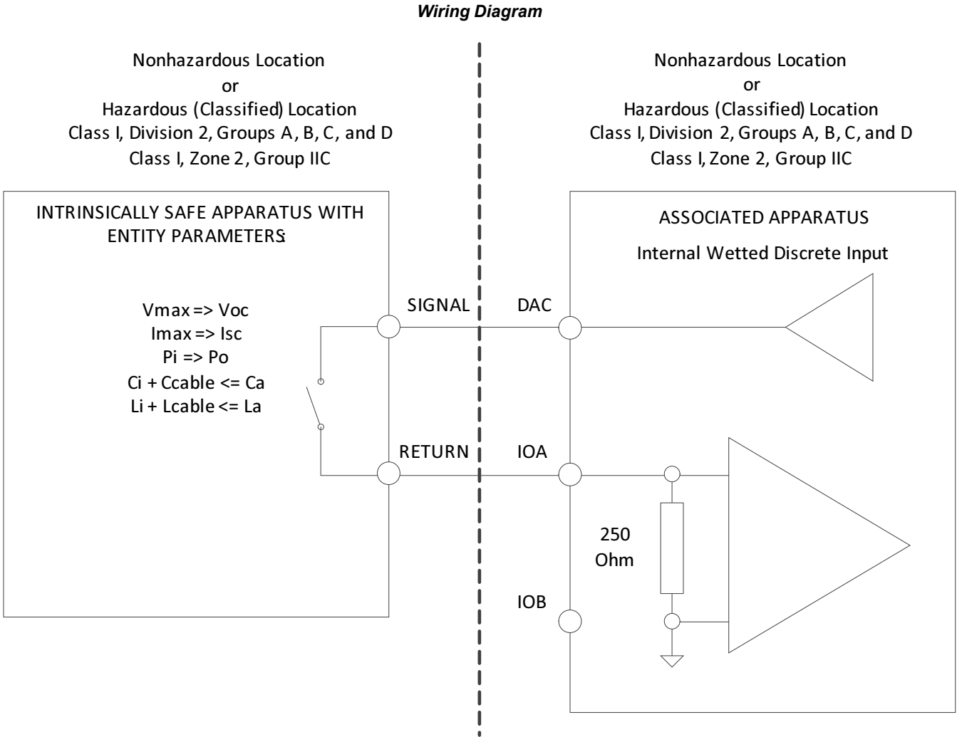
Entity Parameters
